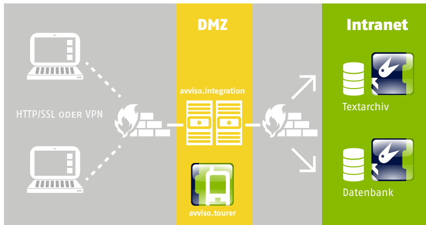
Technisches Systemschema
